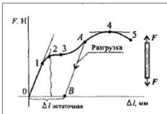
Рисунок 1 - Диаграмма растяжения низкоуглеродистой стали
