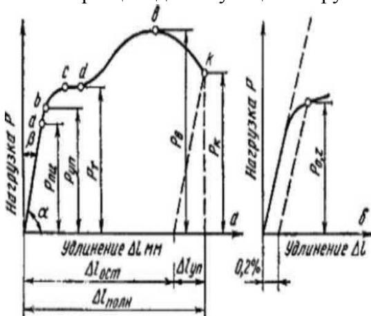
Рис. 2. Диаграмма растяжения
